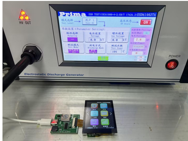
图 7-2 ESD 测试图
