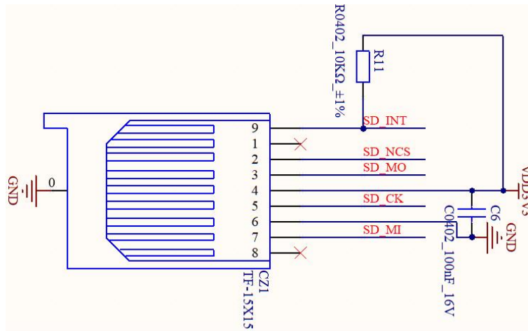
图 6-3 SD 卡座电路示意
