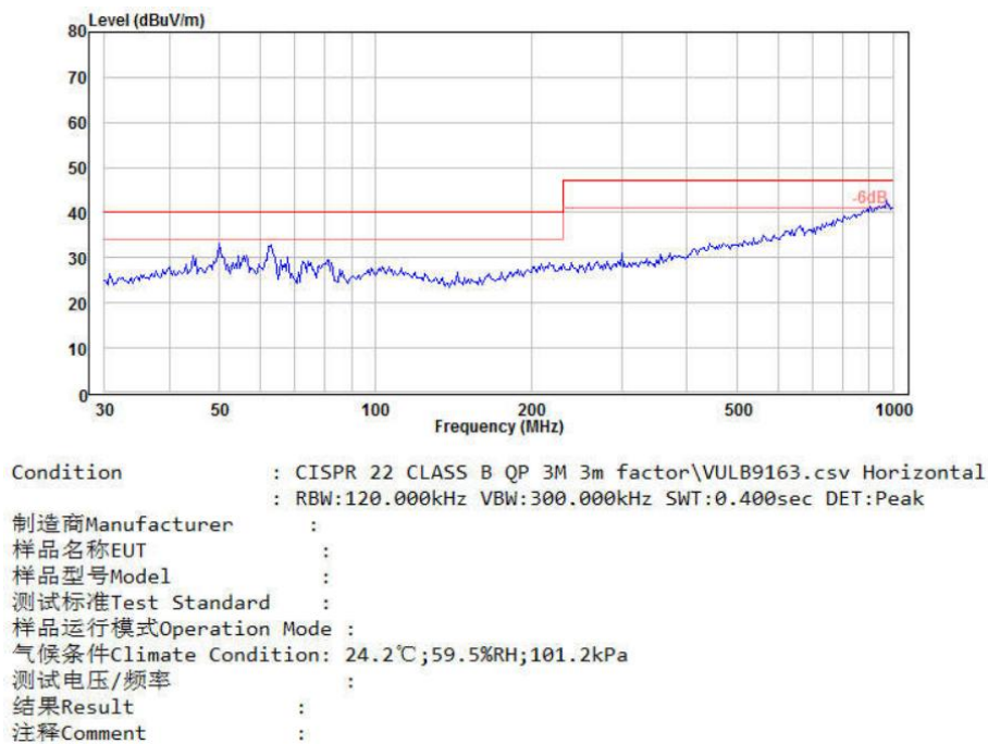
图 7-7 辐射测试垂直方向
