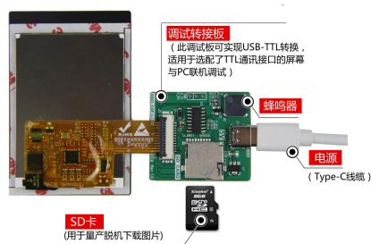
图 1-5 调试工具图
