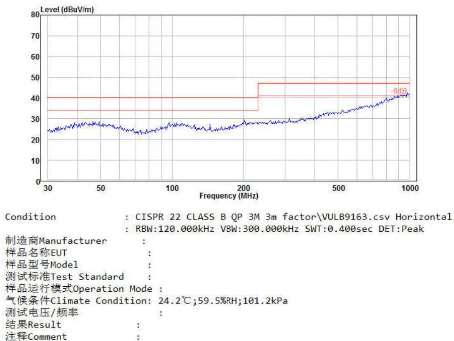
图 7-6 辐射测试水平方向
