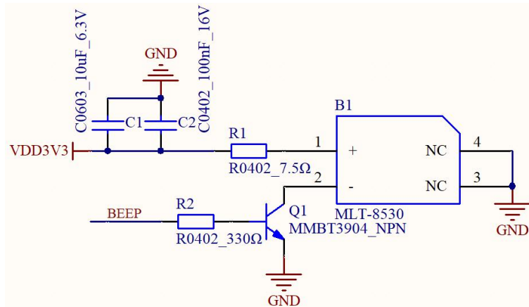
图 6-2 蜂鸣器电路示意
