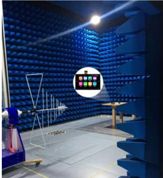
图 7-5 辐射测试图
