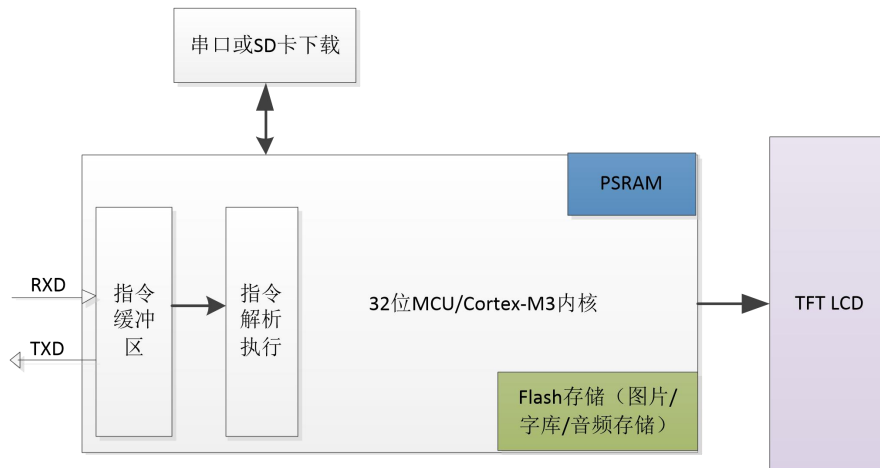
图 12-1 S 系列串口屏内部结构图
